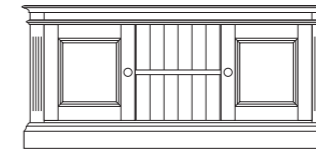
Midi 2 Door TV Unit H 603mm x W 1330mm x D 450mm AFEV280
